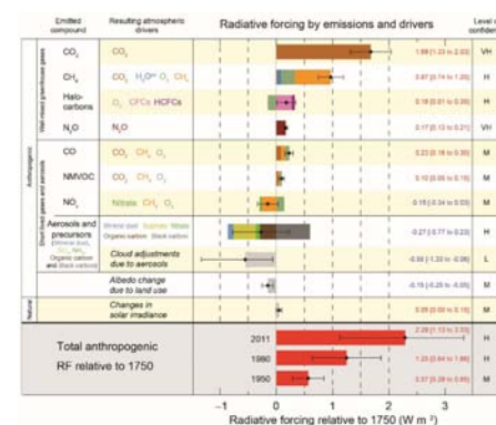
Figuur: Oorzaken van stralingsforcering (IPCC 2013 AR5 SPM)
