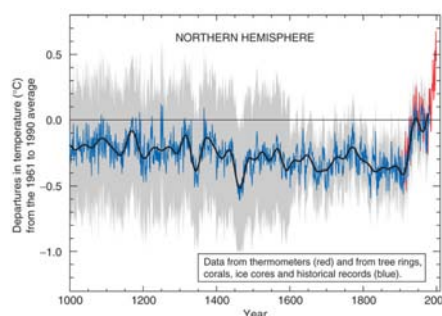
Figuur: De temperatuurafwijking van het afgelopen millennium (IPCC 2001)
